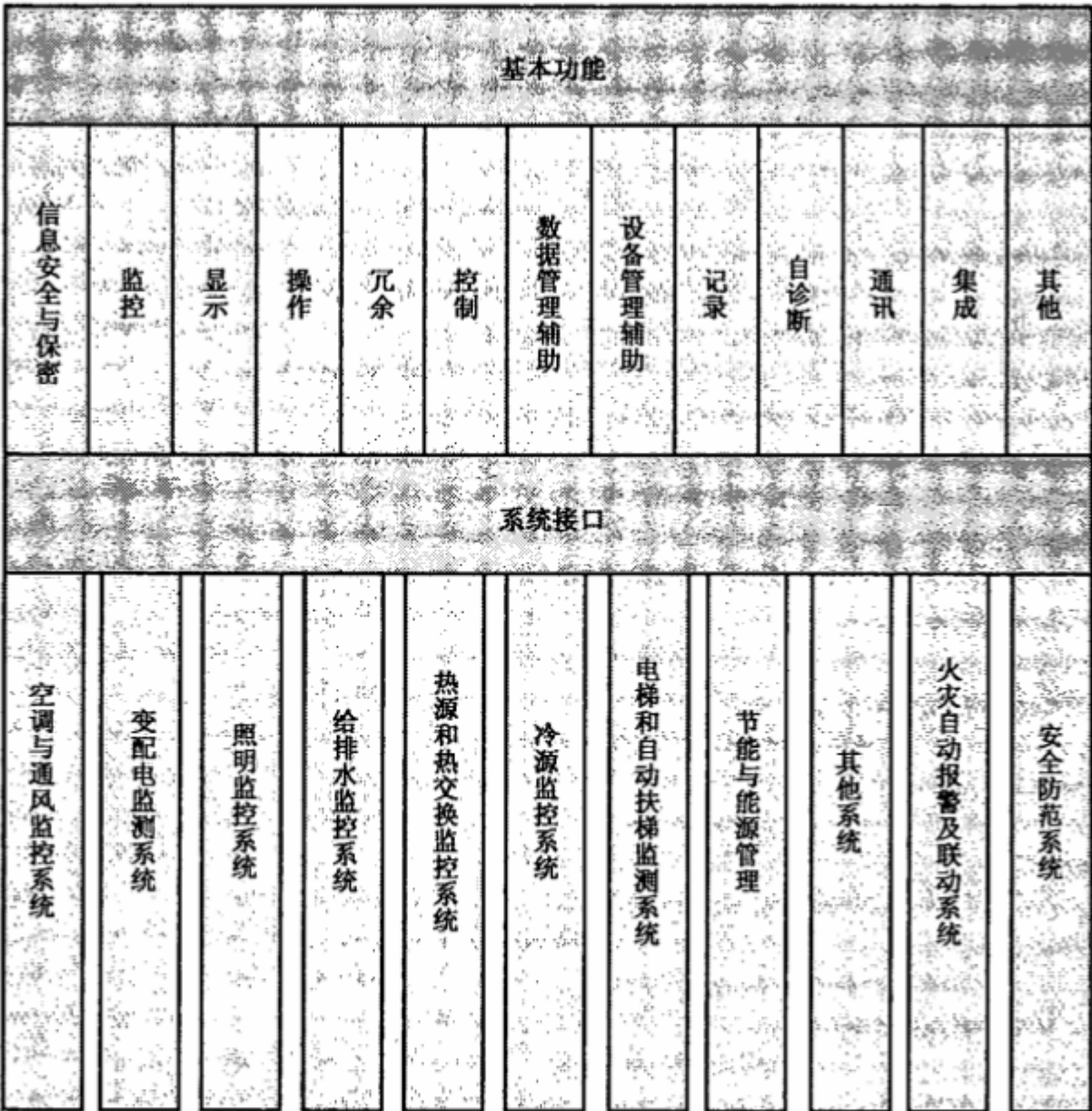
图 1 BACS 框架图
