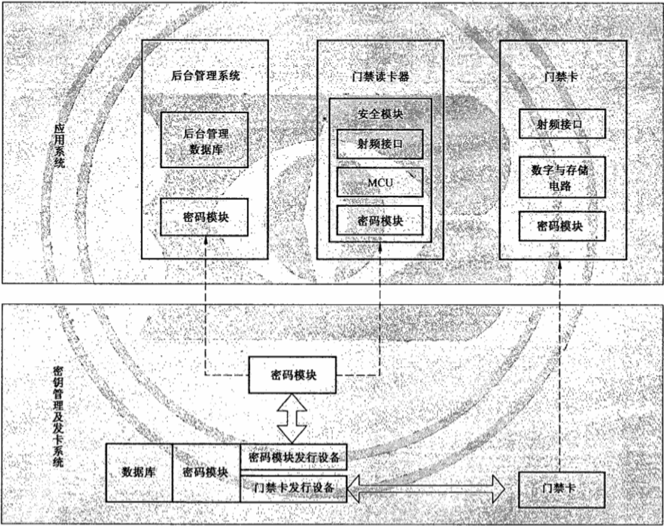
图 C.1 门禁系统中密码应用结构图
