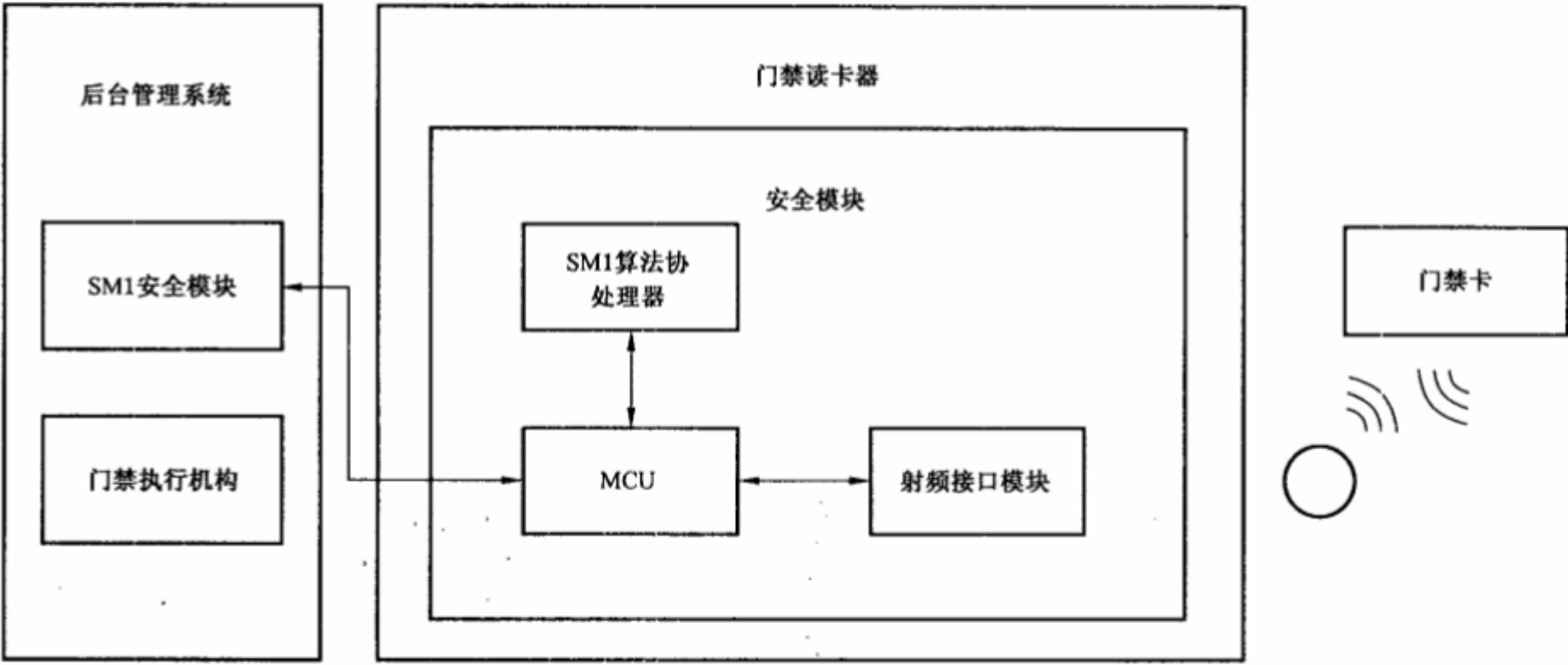
图 C.3 原理图
